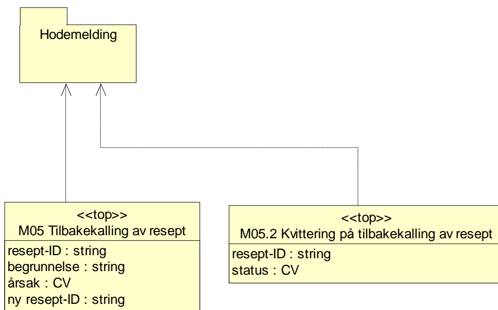
Diagram: M5.2 Kvittering på tilbakekalling av resept
